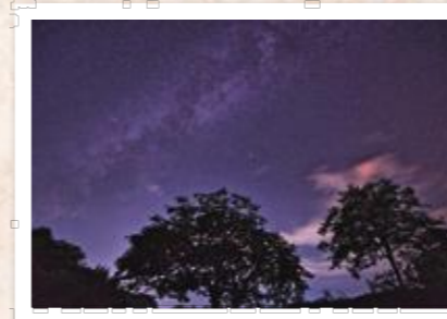
夏の天の川
