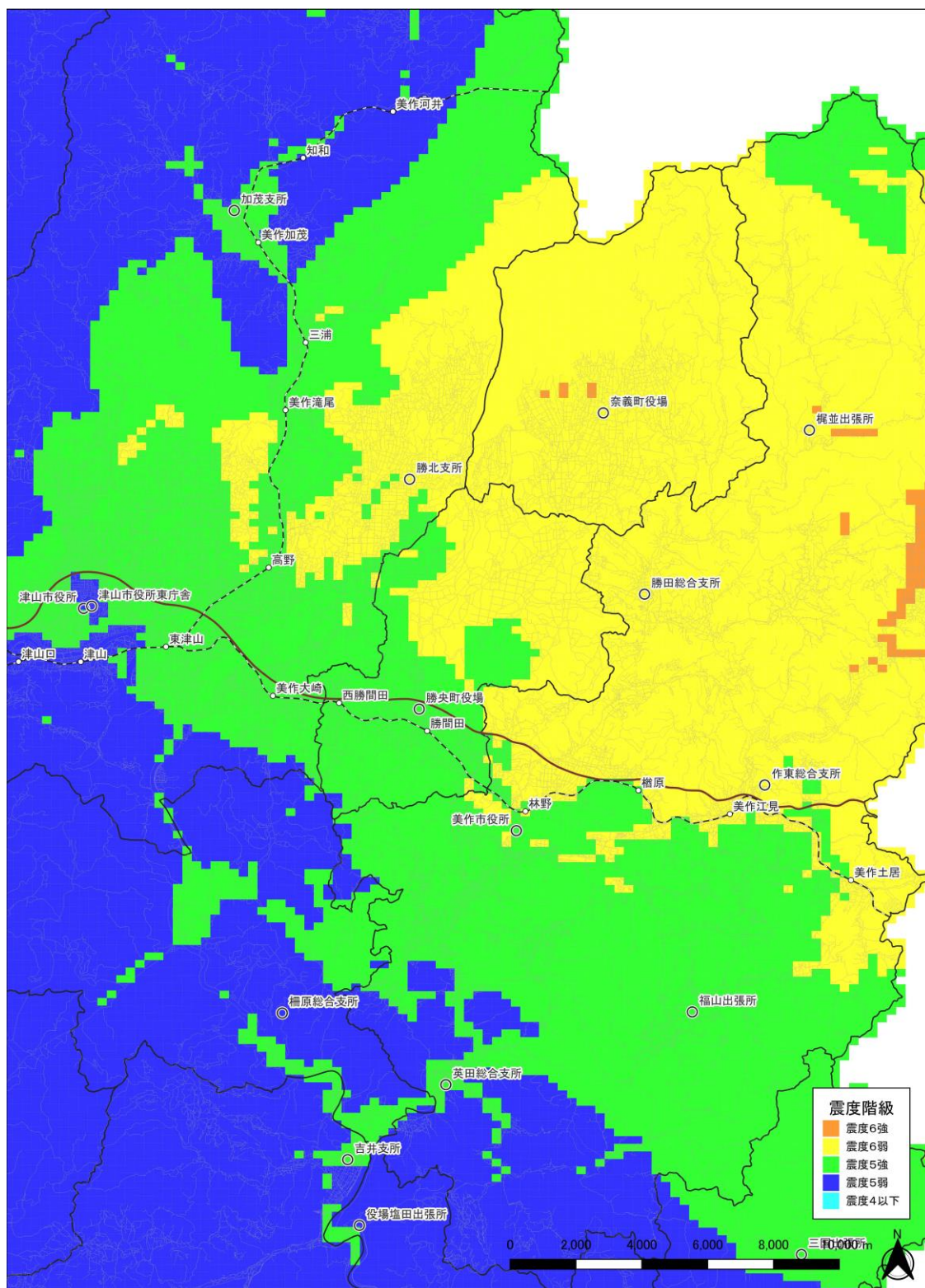
震度分布図
