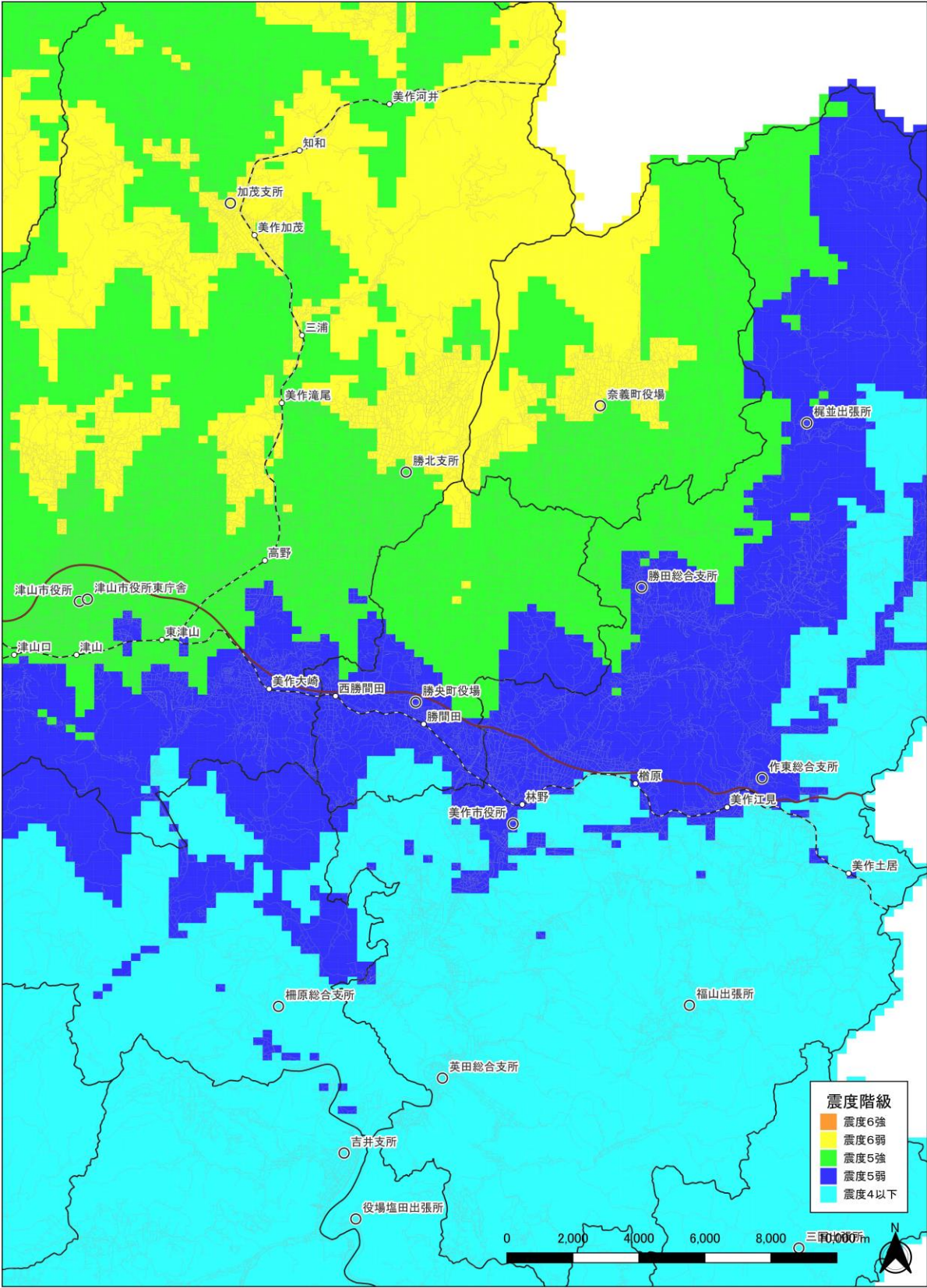
震度分布図
