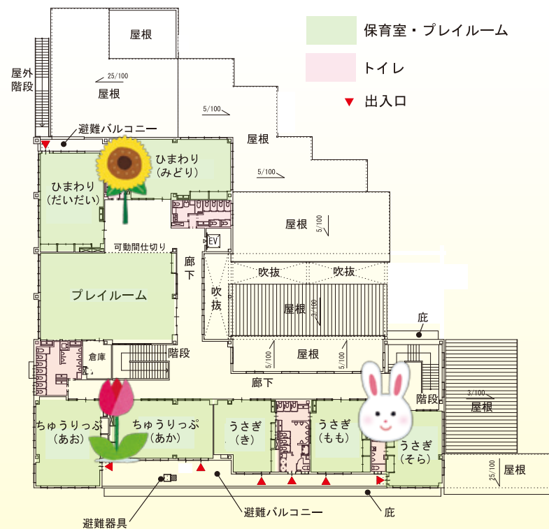
2階平面図
